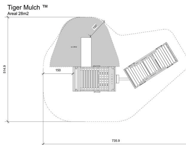
Tiger Mulch™ Areal 28m 2 Det legale område omkring rutsjebane. Samt omkring campingvogn hvis man skulle følge den typisk 150cm som minimum afstand af fald areal.
